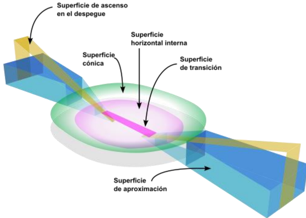
Figura 97. Superficies limitadoras de obstáculos consideradas para la elaboración de los mapas de aeródromo y de obstáculos de aeródromo. Fuente: UNAM.
