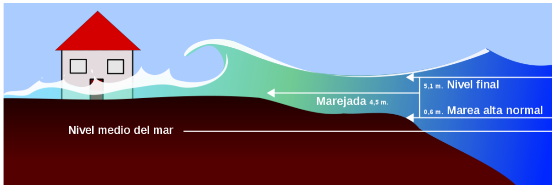
Figura 63. Marea de tormenta. Fuente: (Robbert Simmon, 2017)
