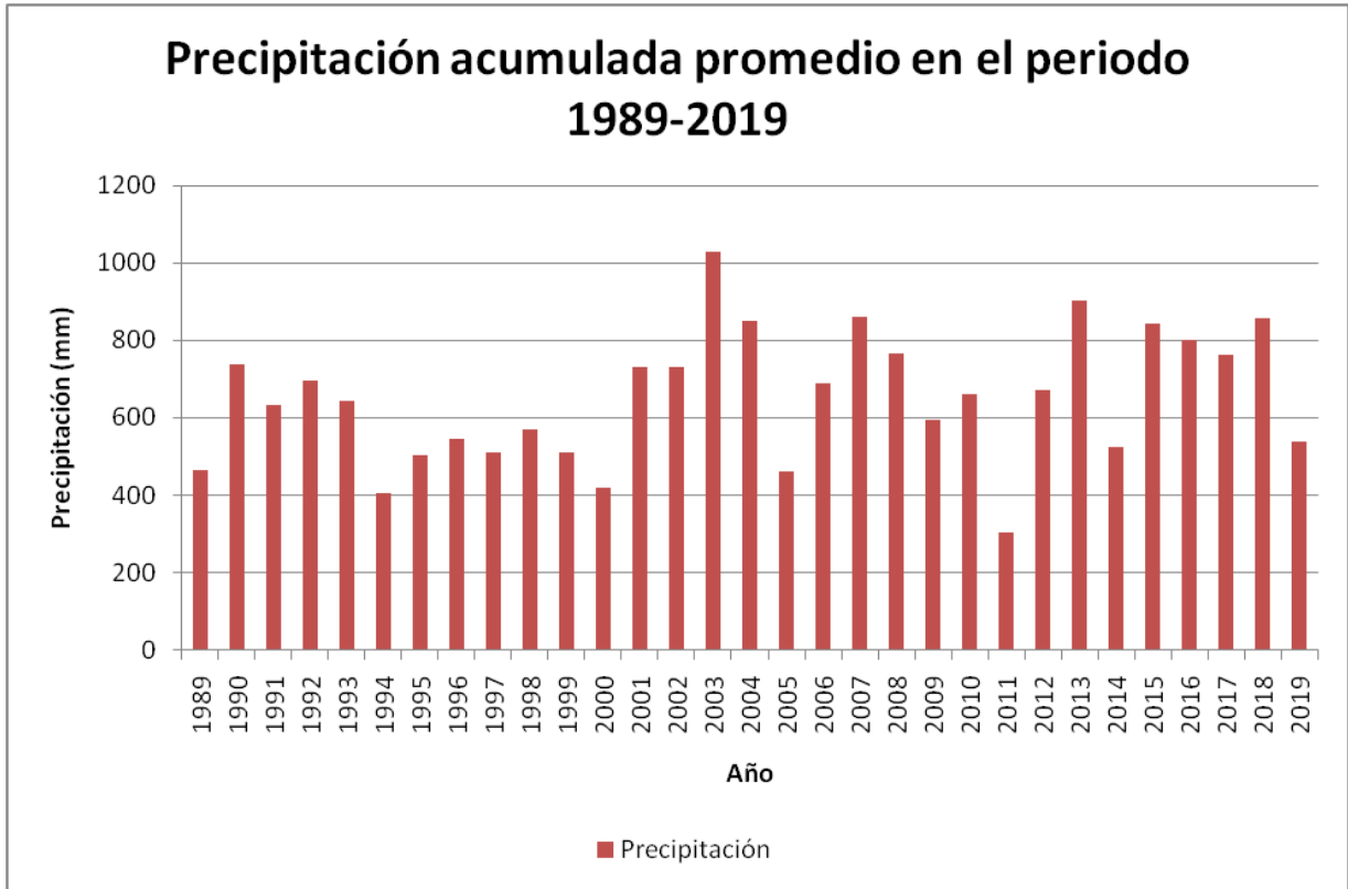
Figura 20. Precipitación Acumulada Promedio
