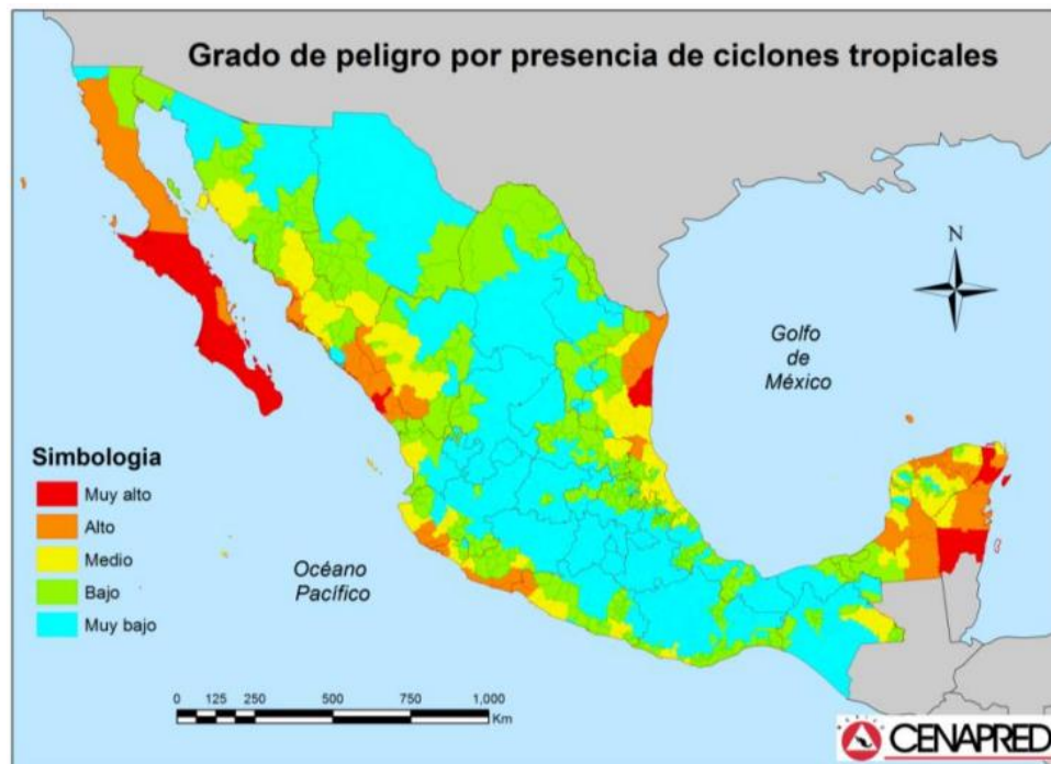
Figura 64. Grado de peligro por presencia de ciclones tropicales. Fuente: (CENAPRED, 2012)
