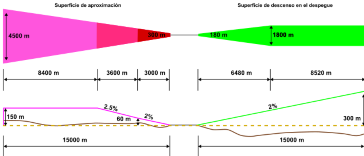
Figura 98. Superficies de aproximación y de ascenso en el despegue. Fuente: UNAM.
