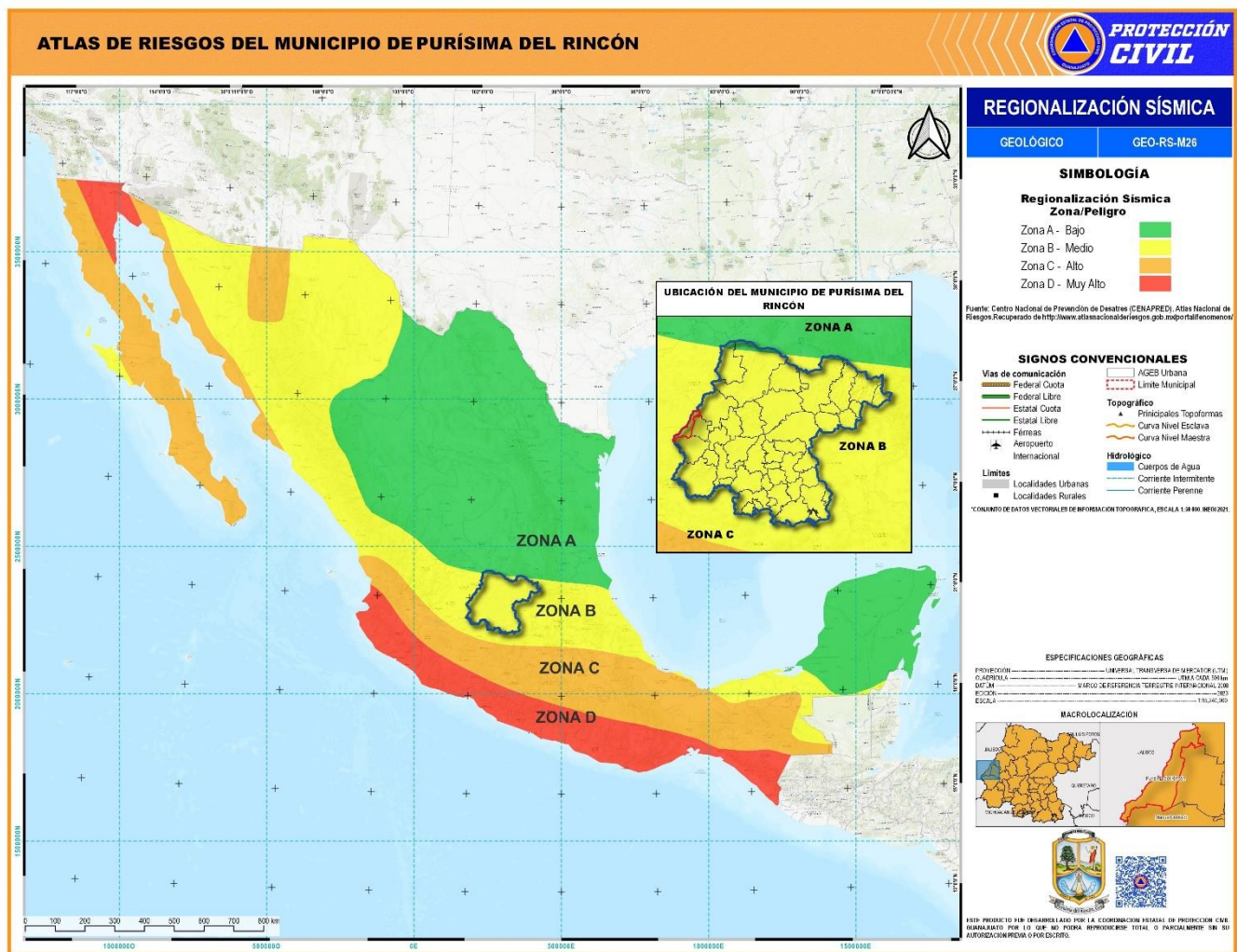
Figura 54. Mapa de regionalización sísmica del Estado de Guanajuato con enfoque a nivel nacional. Fuente: (CEPC)
