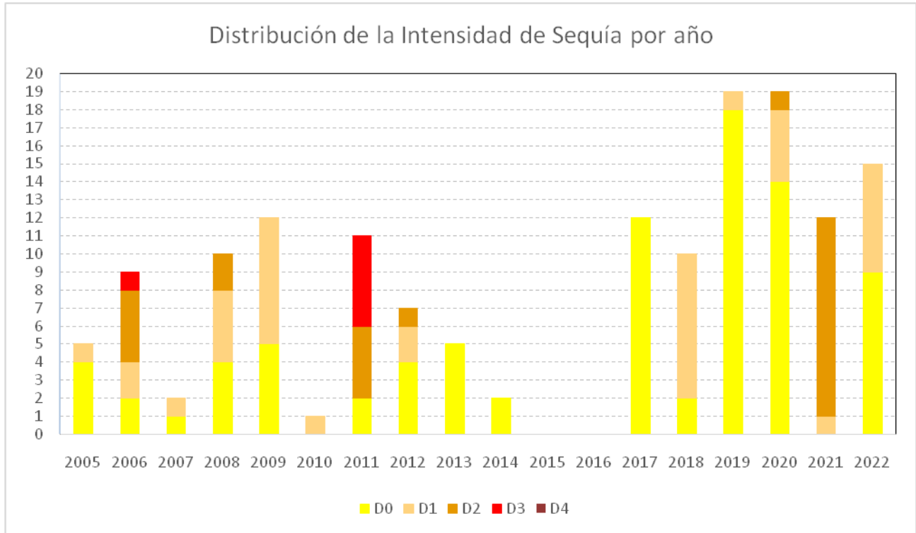
Figura 71. Monitor de Sequía para el Municipio de Purísima del Rincón
