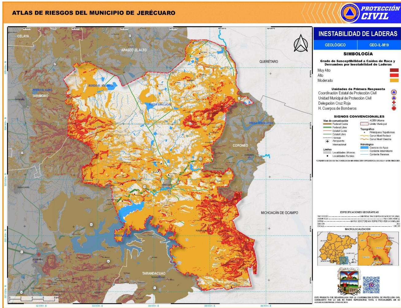
Figura 51. Mapa de susceptibilidad por inestabilidad de laderas del municipio de Jerécuaro, Gto.
