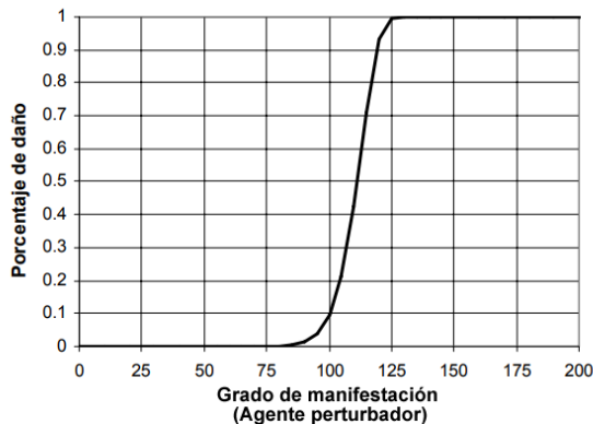
Figura 40. Función de vulnerabilidad para elemento con falla frágil. Fuente: CENAPRED
