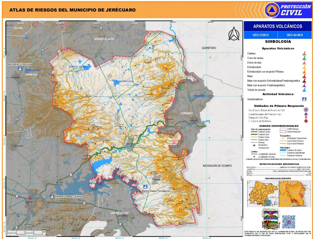
Figura 61. Mapa de estructuras volcánicas y sitios de manifestaciones geotérmicas del municipio de Jerécuaro, Gto.
