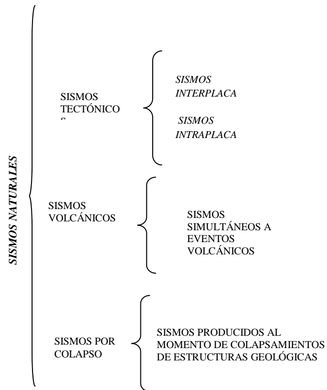
Figura 1. Clasificación de los Sismos Naturales
