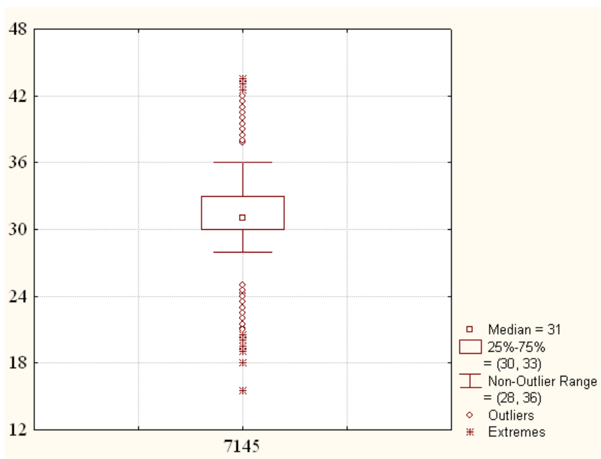
Fig.VII. Boxplot de temperatura máxima para la estación 7145, San Francisco II Chiapas.
