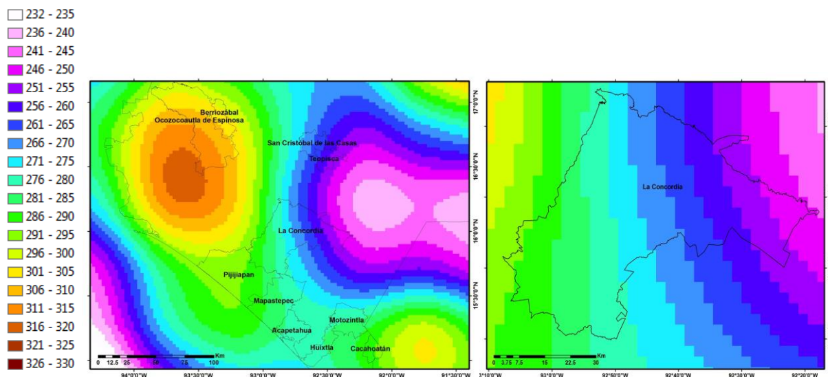
Fig. IV Número de descargas eléctricas por km 2 registradas anualmente por el sensor LIS de la NASA, como indicador de actividad eléctrica sobre el estado de Chiapas y el municipio de La Concordia.
