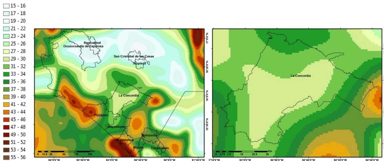
Fig. 12 Percentil 90% de la precipitación diaria (mm) en el estado de Chiapas y en el municipio de La Concordia.
