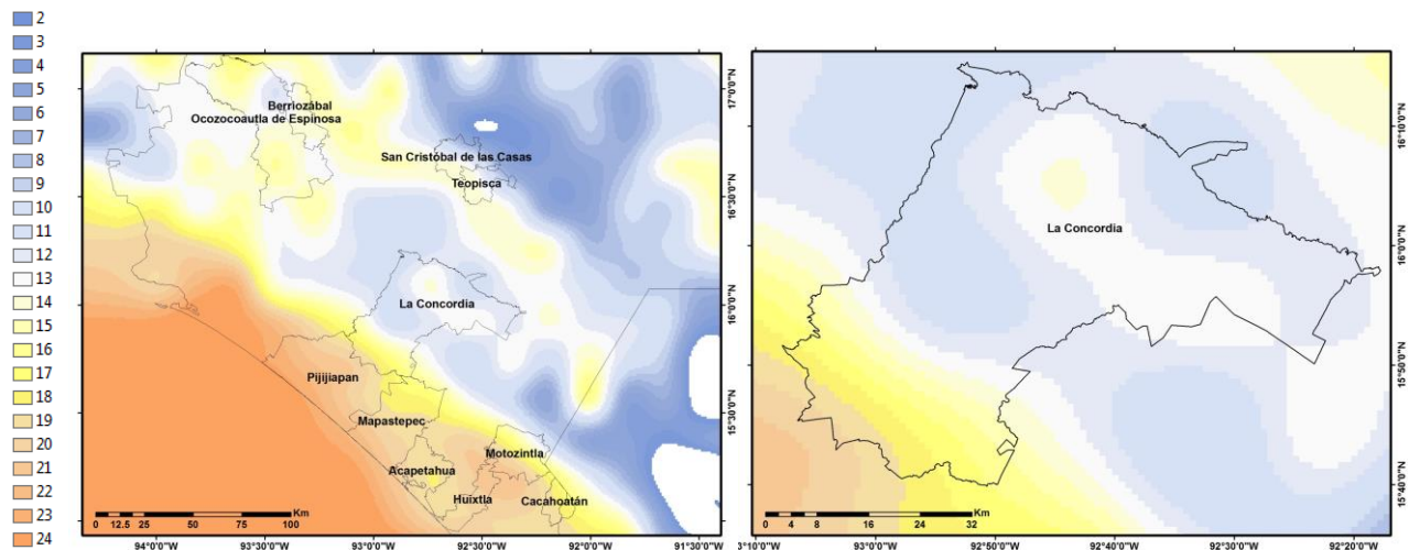
Fig. IX. Temperatura mínima (°C) percentil 10%, para los meses más fríos (diciembre, enero y febrero) en parte de Chiapas y en el municipio de La Concordia.
