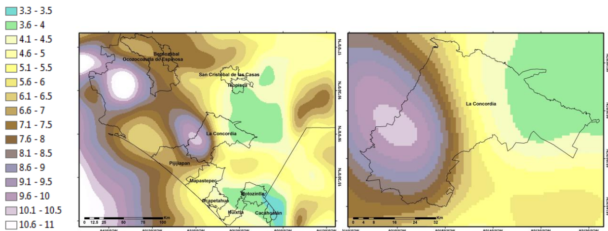
Fig. XI. Percentil 90 de la magnitud de viento (m/s) en el estado de Chiapas y en el municipio de La Concordia.
