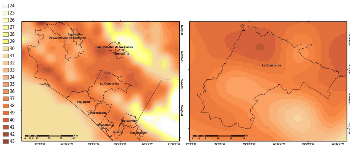
Fig. VI. Percentil 90% de la temperatura máxima (°C) para los meses más cálidos (marzo, abril y mayo) en parte de Chiapas y en el municipio de La Concordia..
