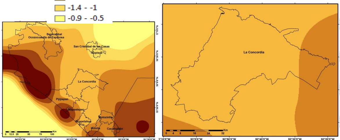
Fig. V. Severidad de la sequía meteorológica en Chiapas y La Concordia durante el verano (mayo-octubre) de 1972,1977 y 1986, de acuerdo a valores del SPI-6.
