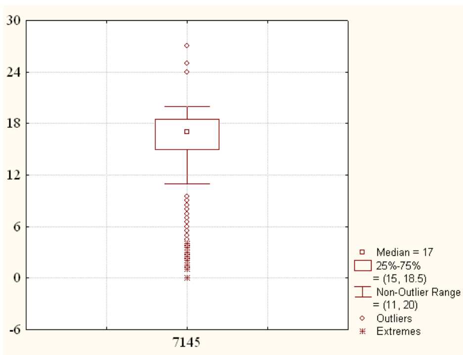
Fig. X. Boxplot de temperaturas mínimas en La Concordia de Chiapas.
