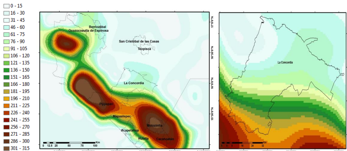
Fig. 14 Precipitación ocurrida en el estado de Chiapas el 4 de octubre de 2005 bajo los efectos del huracán Stan
