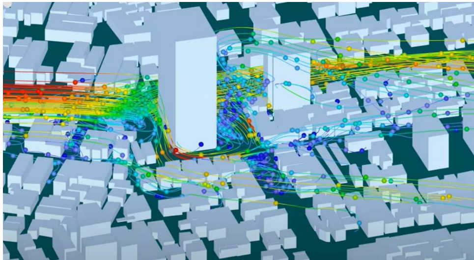
Figura 40. Comodidad del viento en zonas peatonales y alrededor de edificios. Fuente: Rwind Simulation.
