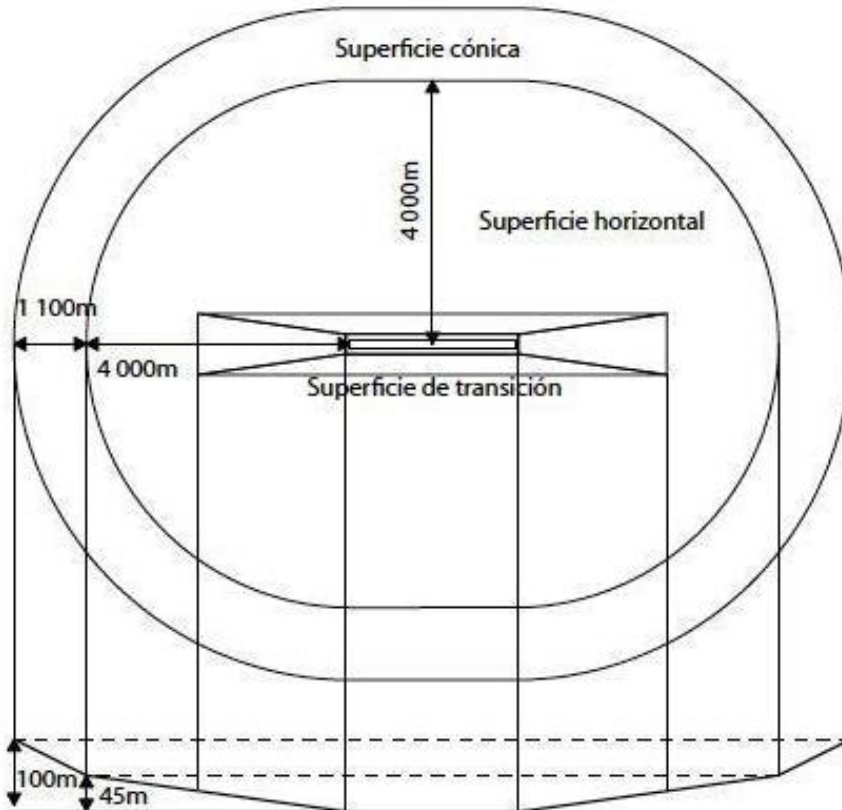
Figura 100. Vista en planta y de perfil de las superficies de transición, horizontal interna y cónica. Fuente: UNAM.
