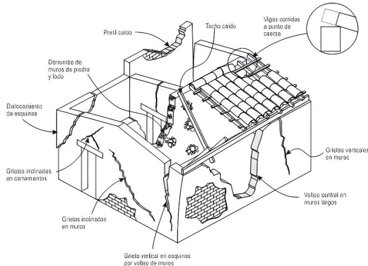
Figura 43. Daños comunes en viviendas rurales. Fuente: (Flores et al., 2001)
