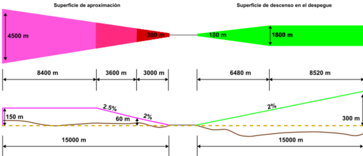
Figura 99. Superficies de aproximación y de ascenso en el despegue. Fuente: UNAM.
