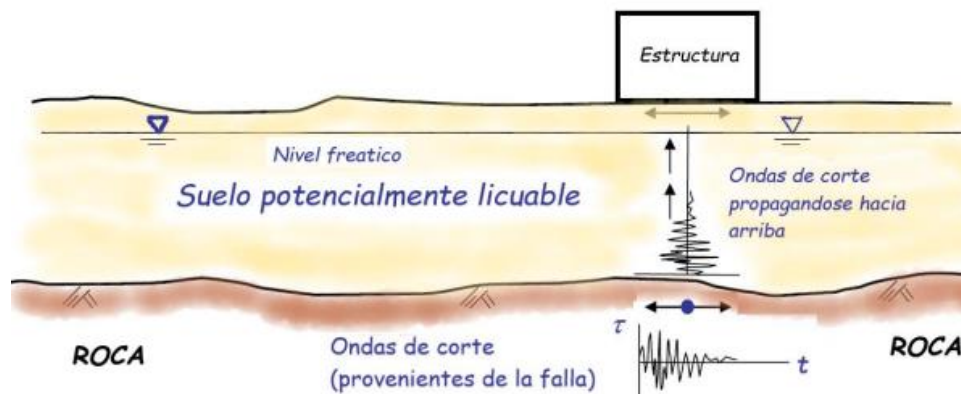
Figura 54. Esquema mostrando la generación del fenómeno de licuación sísmica. Fuente: (Pando, 2020)
