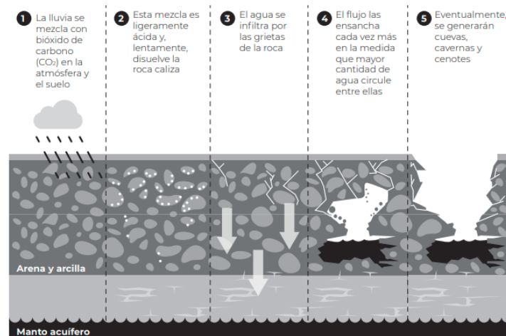
Figura 55. Etapas de formación de cavidades. Fuente: (CENAPRED)
