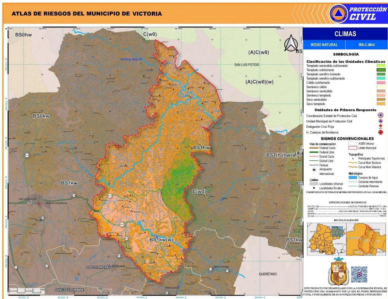
Figura 17. Clasificación del Clima en el municipio de Victoria, Gto.
