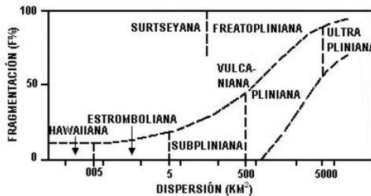
Figura 61. Distancia alcanzada por la ceniza desde el centro de emisión de acuerdo con el porcentaje de fragmentación y tipo de erupción. Fuente: CENAPRED.
