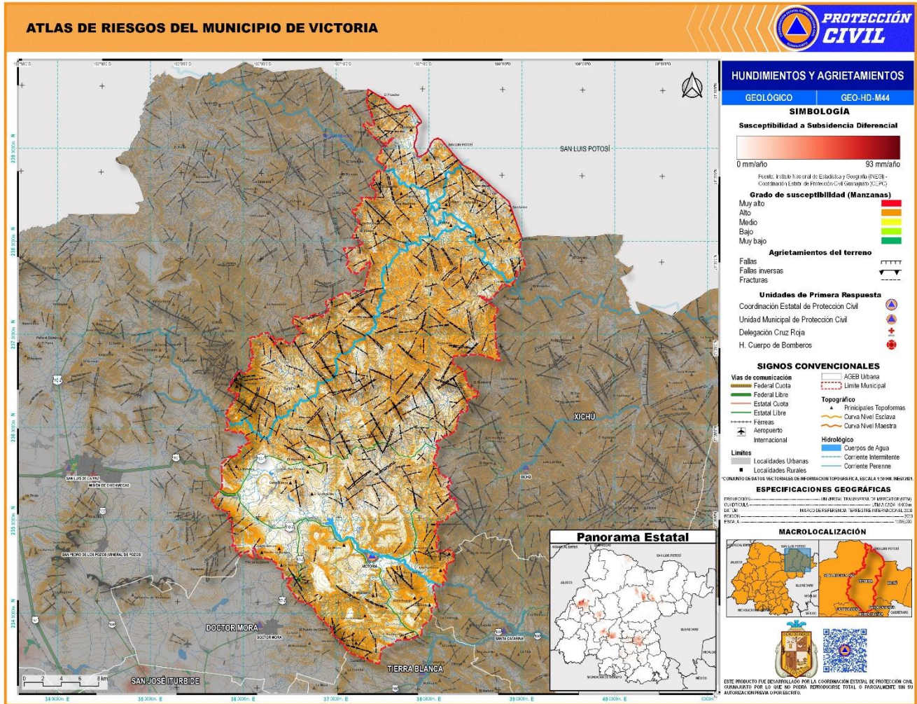
Figura 63. Mapa de Agrietamiento del terreno en el municipio de Victoria, Gto. Atlas Estatal de Peligros y Riesgos.
