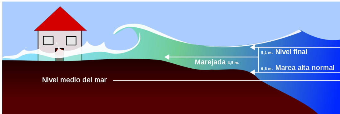
Figura 64. Marea de tormenta. Fuente: (Robbert Simmon, 2017)
