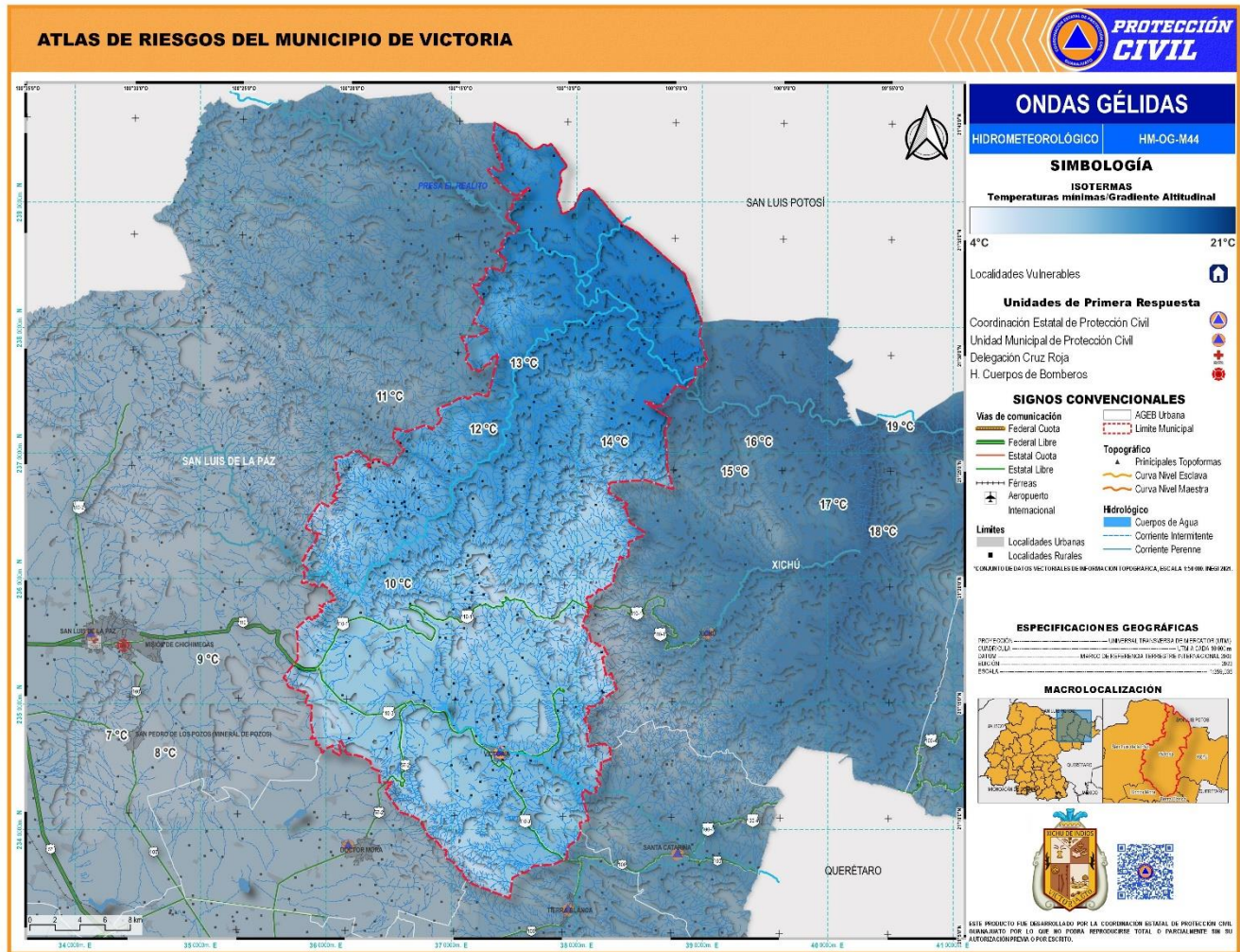
Figura 75. Mapa de Ondas Gélidas en el municipio de Victoria, Gto. Fuente: CEPC, GTO
