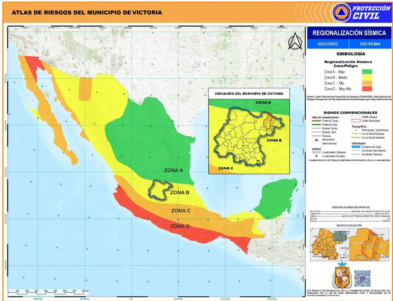
Figura 56. Mapa de regionalización sísmica del Estado de Guanajuato con enfoque a nivel nacional.
