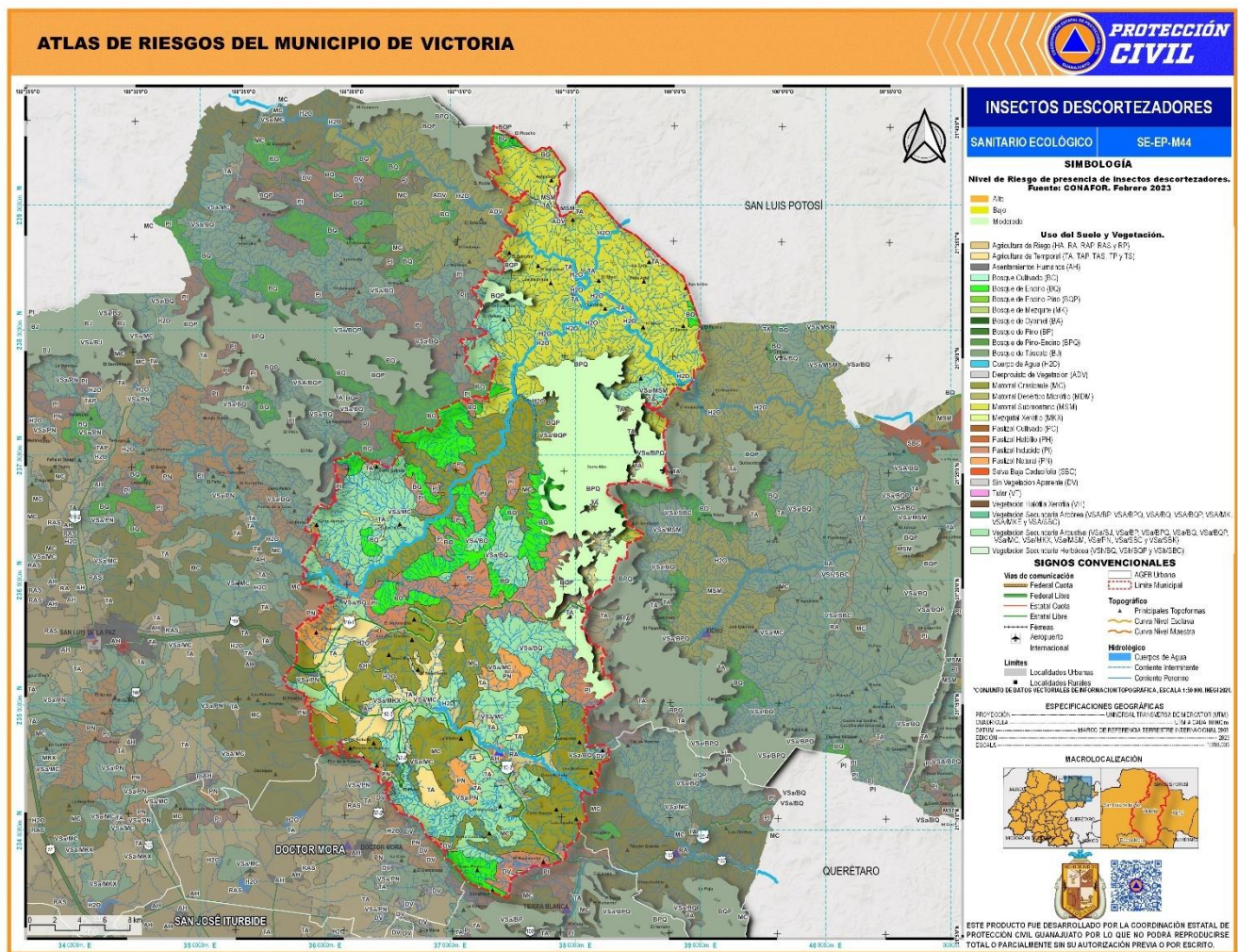
Figura 89. Mapa de Insectos Descortezadores.
