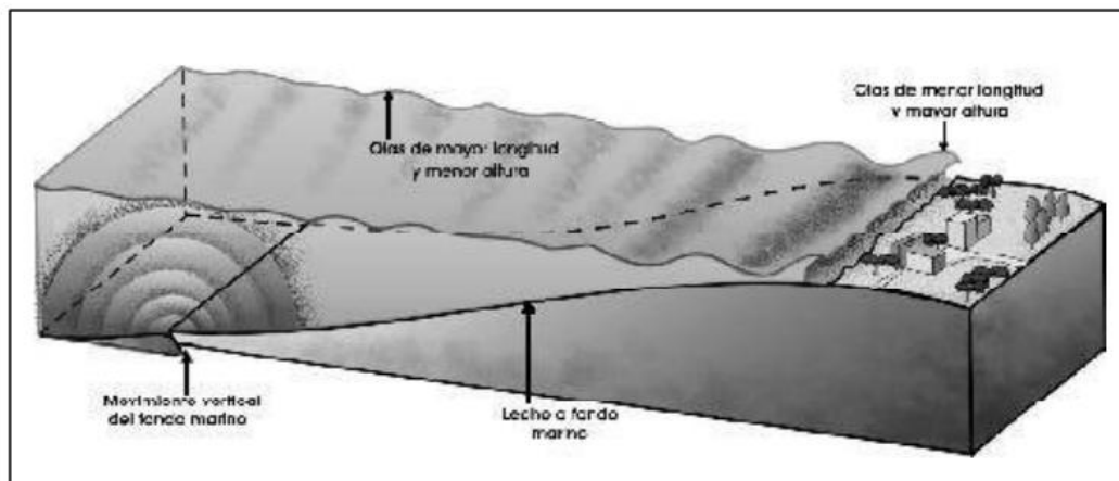
Figura 60. Generación, propagación y arribo a la costa de un tsunami. Fuente: (Fascículo “Tsunami”, 2005).
