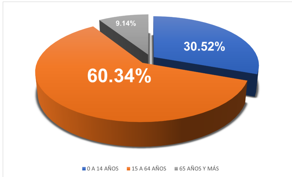
Figura 26. Distribución de la población por rango de edad en el municipio de Victoria. Fuente: (INEGI, 2020a)
