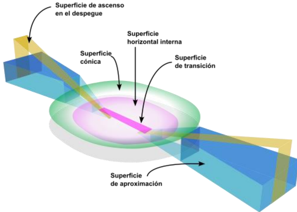
Figura 103. Superficies limitadoras de obstáculos consideradas para la elaboración de los mapas de aeródromo y de obstáculos de aeródromo. Fuente: UNAM.
